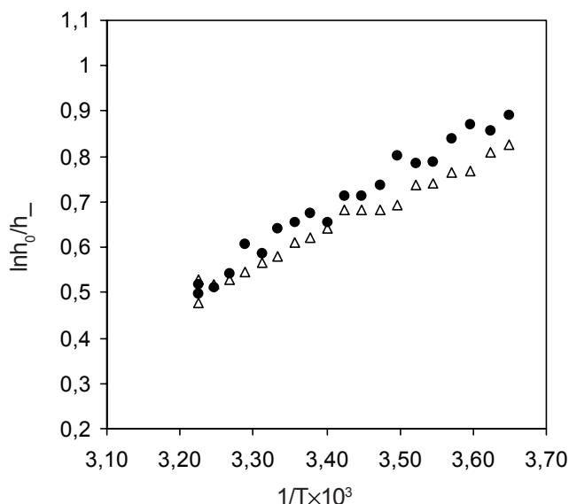
Рис. 4. Залежності Ареніуса параметра рухливості зонда TEMPON у цитозолі еритроцитів: ● – нативних, △ – після інкубації з фракцією менше 5 кДа ЕПЛ, що зберігалася при -20^{\circ}\text{C} .
